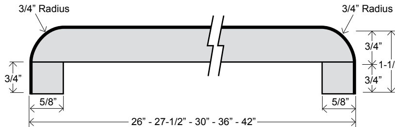
BAR TOP PTB 26 PTB 27-1/2 PTB 30 PTB 36 PTB 42
