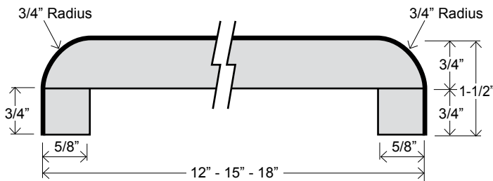
BAR TOP PTB 12 PTB 15 PTB 18
